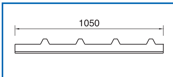
Profilo chiudigrecia in acciaio preverniciato
