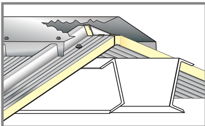
Montaggio colmo
