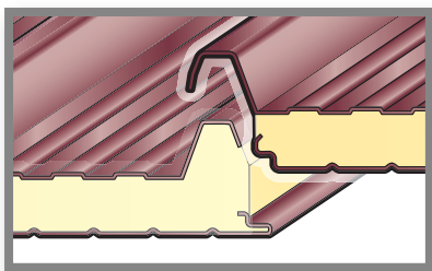
sovrapposizione laterale di una greca
